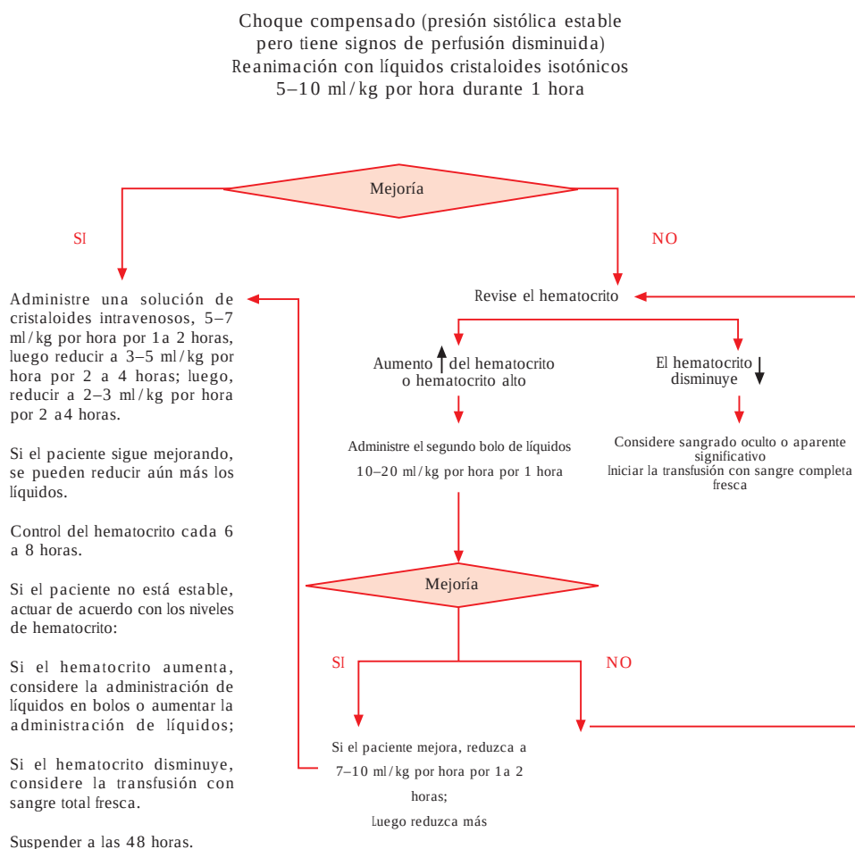
Figura 2.2 Algoritmo para el manejo de líquidos en el choque compensado
